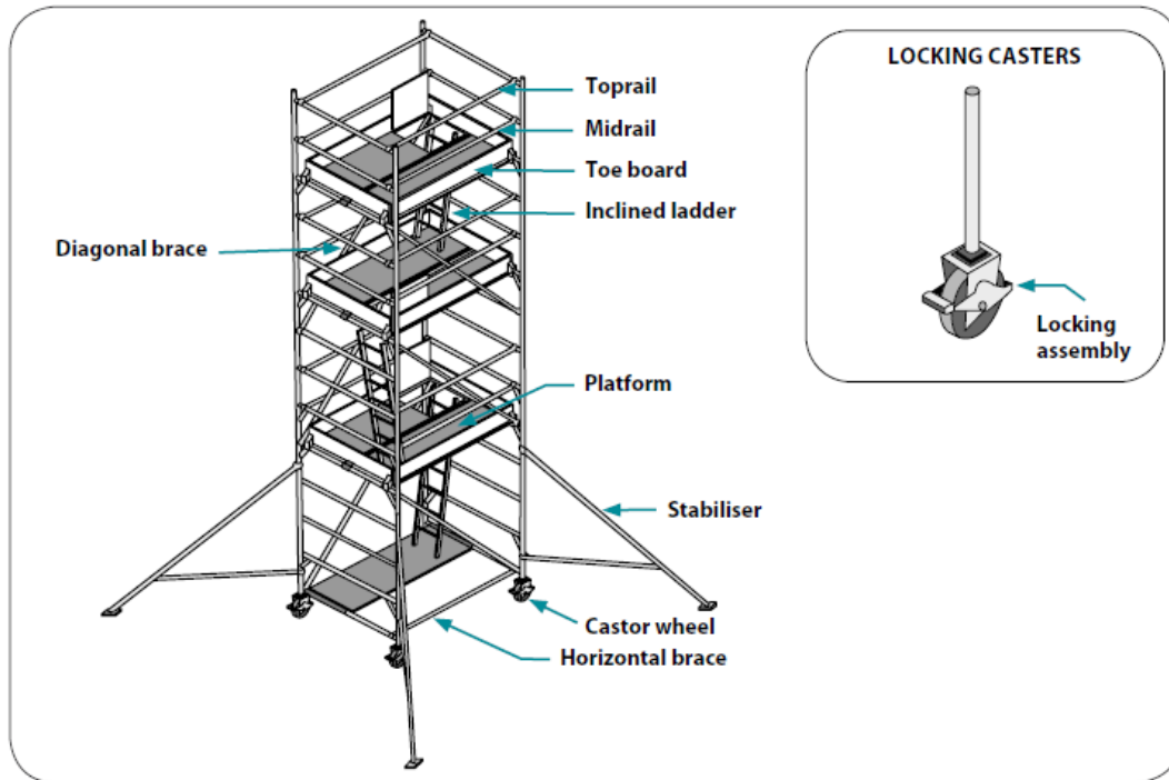
圖 28 移動塔式腳手架
