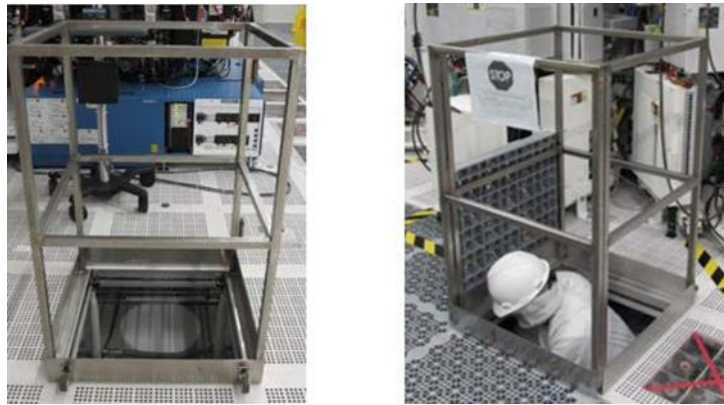
圖 20 單地磚路障
