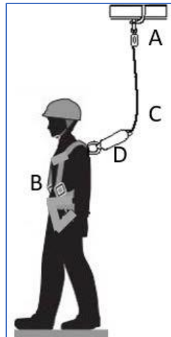
圖 4 防跌落系統
